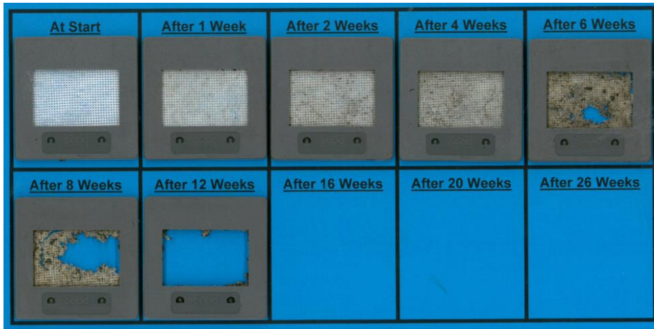
ホームコンポスト環境下（28℃）での崩壊予備試験結果
