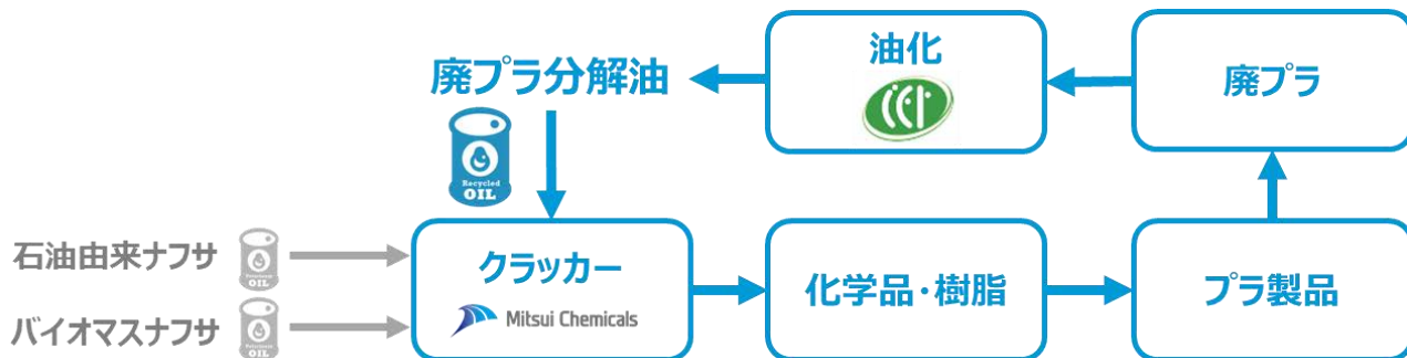
【ケミカルリサイクルのフロー図】
