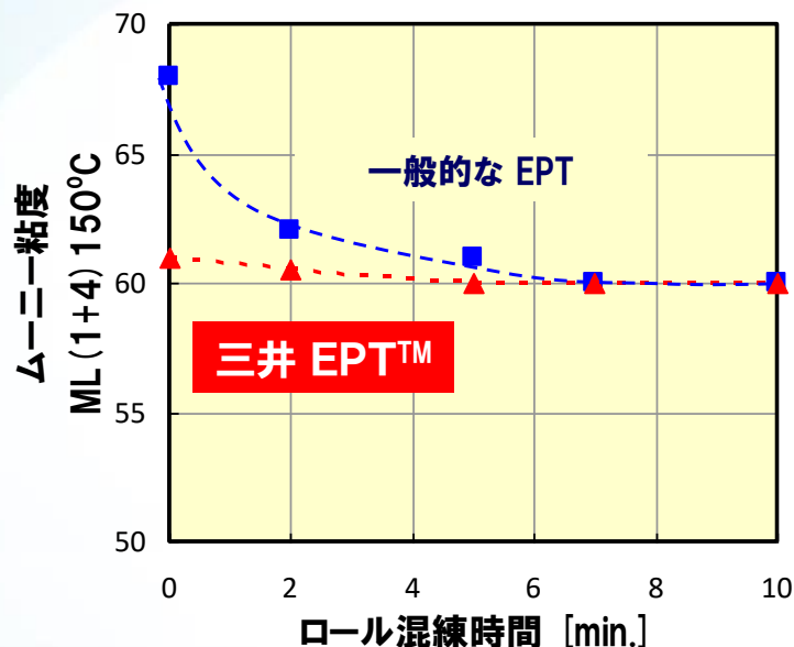
EPTの粘度変化
