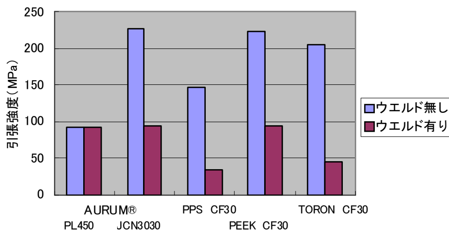
図-1:ウエルド有り、無しの引張強度の変化
