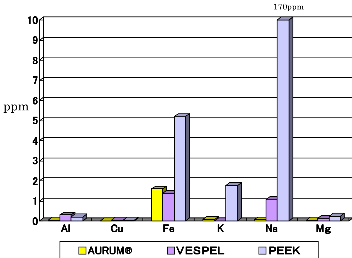
図-1：金属不純物分析データ
